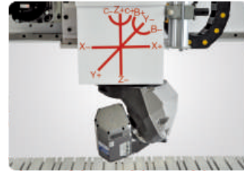
İtalyan menşeli orijinal mil
