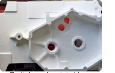
Elyaf kalıp ve ahşap kalıp işleme
