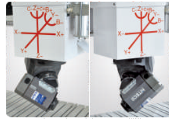
Beş yönde serbest işleme özelliği
