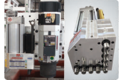
Otomatik takımlı mil + 9V delme ünitesi
