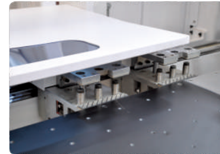
Çift tutuş sistemiyle yüksek hassasiyetli konumlandırma
