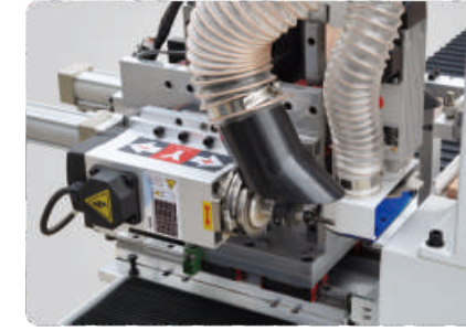
İki kafalı model, iki kafa + testere bıçağı seçeneği ve özel bağlantı elemanlarını destekler
