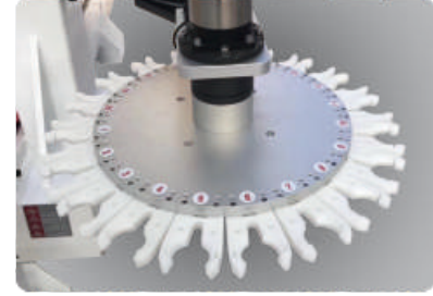
Opsiyonel 20 servo bıçaklı otomatik değişirme sistemi
