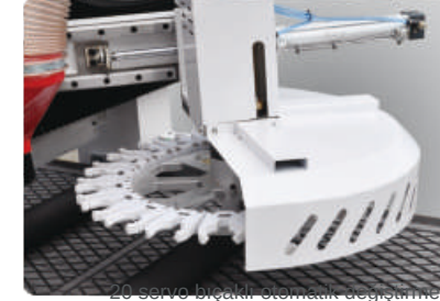
20 servo bıçaklı otomatik değişim özelliği
