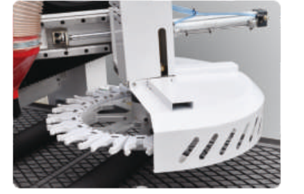
20 servo bıçaklı otomatik değiştirme sistemi
